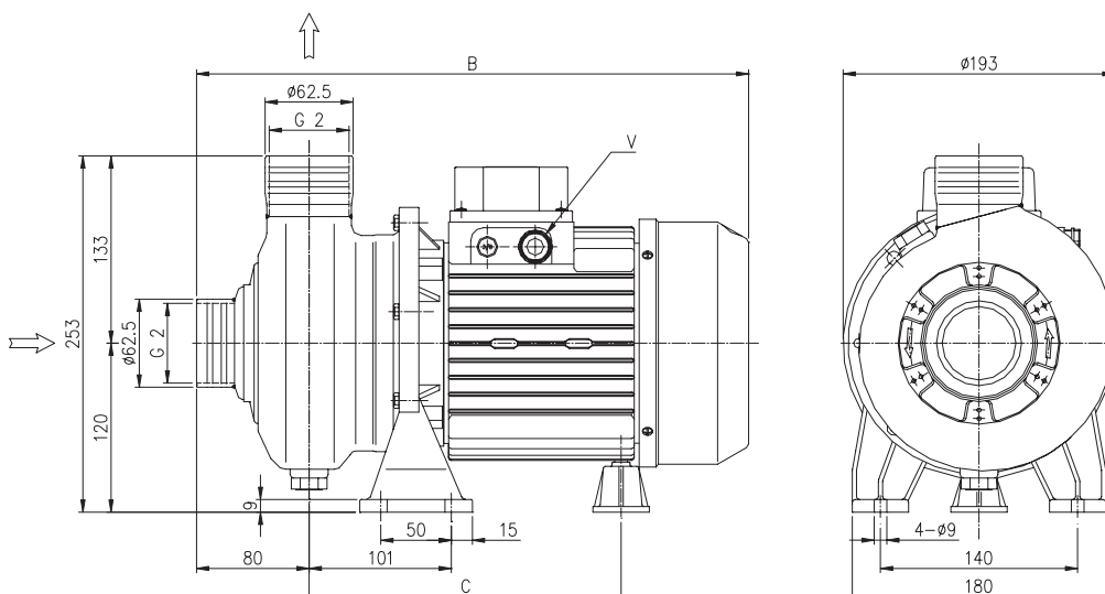
TABULKA ROZMĚRŮ
