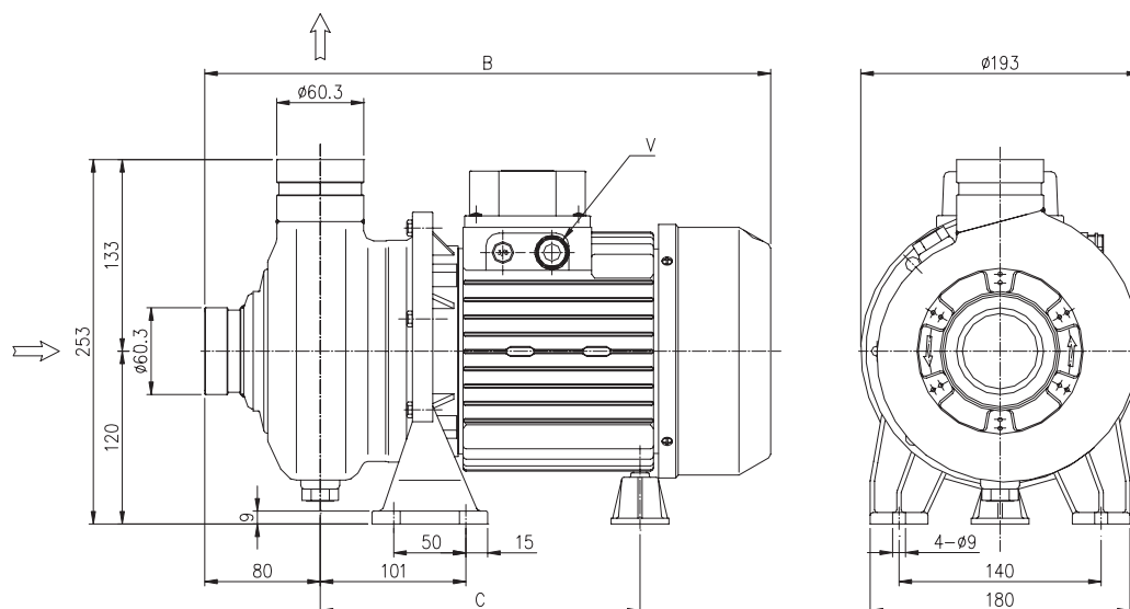
TABULKA ROZMĚRŮ
