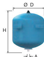
33 litrů s upevňovacími úchyty (pohled zezadu)
